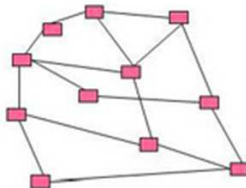
Мультиагентная система
