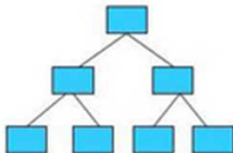
Традиционная (иерархическая)
